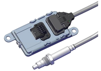
氮氧传感器 NOx Sensor
